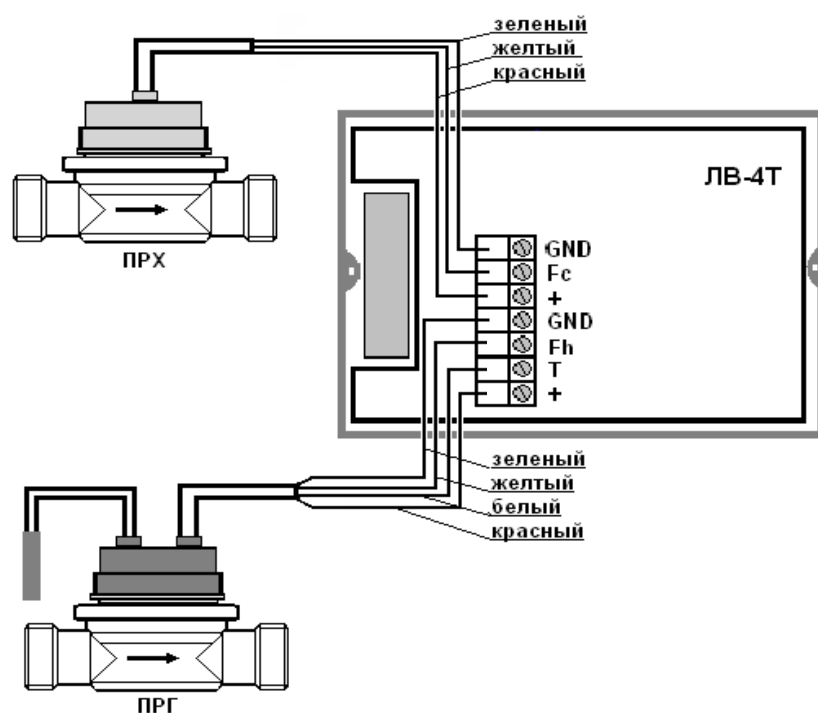
Рисунок 6.3 – Схема электрического соединения счетчика ЛВ-4Т
