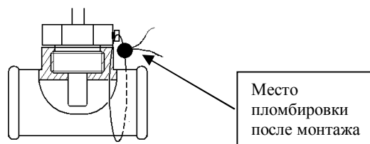
Рисунок 6.1 – Пломбировка датчика температуры после монтажа
