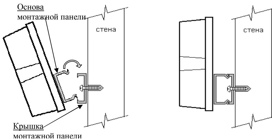
Рисунок 6.4 – Монтаж вычислителя ЛВ на стене
