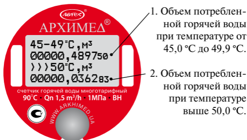
Рисунок 6- Выводимые значения в расширенном режиме индикации.
