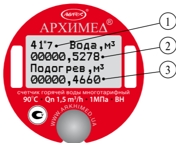
Рисунок 3- Выводимые значения в рабочем режиме индикации.
