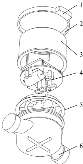
Рисунок А.1- Порядок разборки счетчика.
